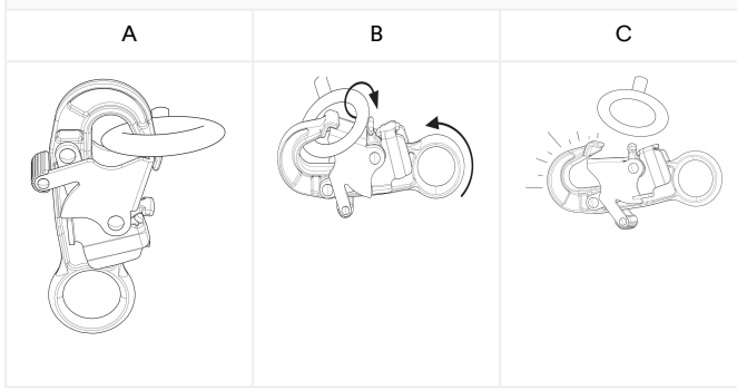
그림 3 - 커넥터 호환성
